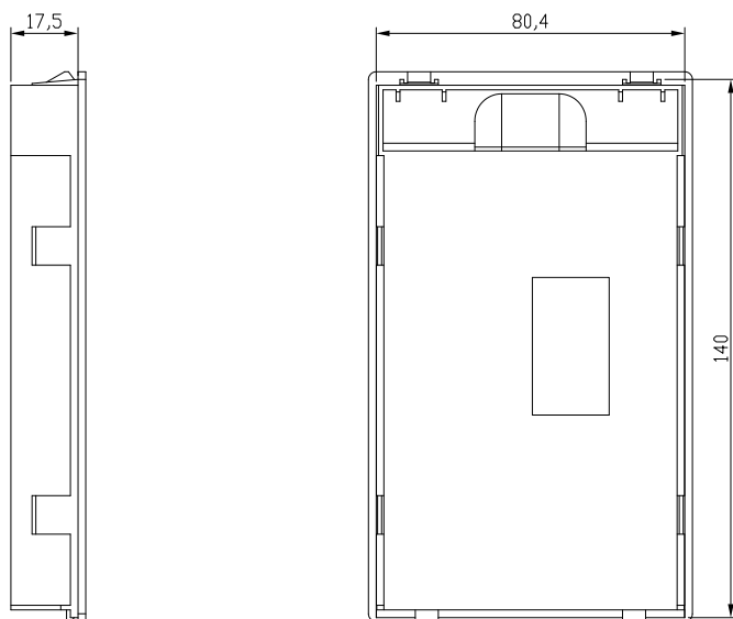
图 1-4 外引键盘支架外形尺寸图 (单位 mm)
