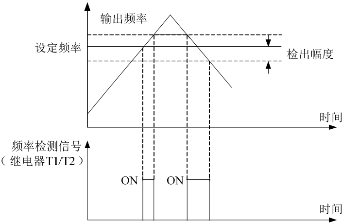
图 5-18 FDT 电平示意图
