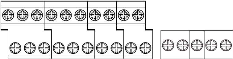
图 2-5 控制板端子示意图
