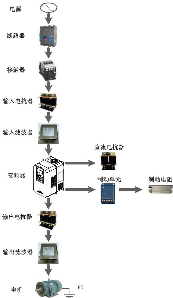
图 2-1 产品外围元器件的标准配置图
