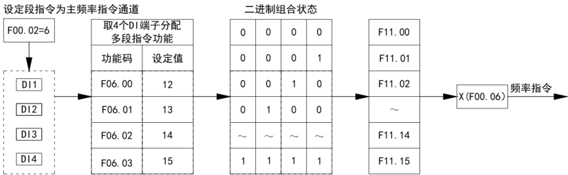
图 5-10 多段速模式的设置
