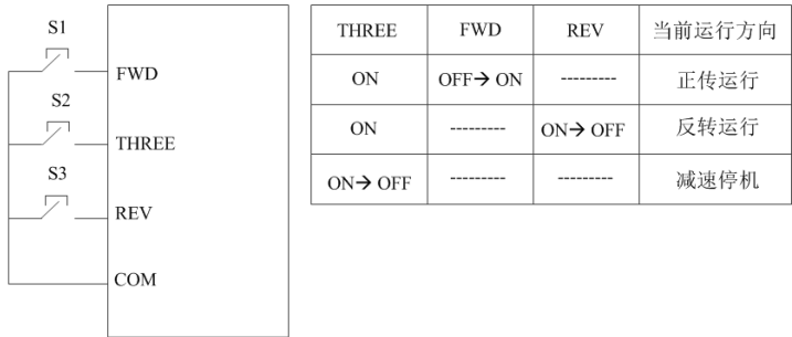
图 5-3 三线式控制 1
