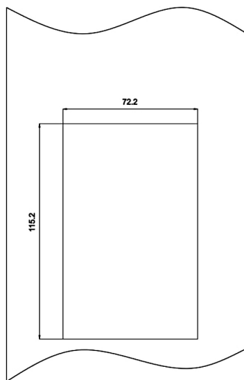
图 1-5 操作面板本体外引开孔尺寸图
