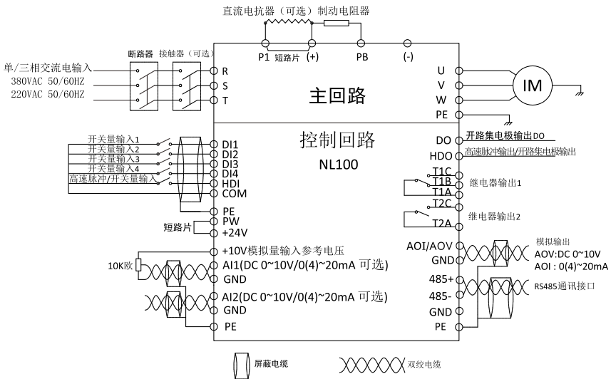
图 2-2 标准接线图
