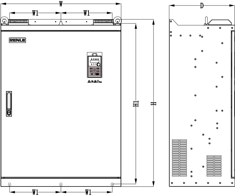
d) 适用于 C7,C8 机箱
