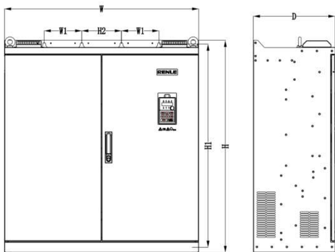
e) 适用于 C9 机箱
