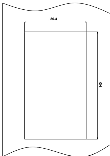
图 1-6 操作面板支架外引开孔尺寸图
