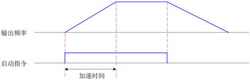
图 5-13 直接启动时序图
