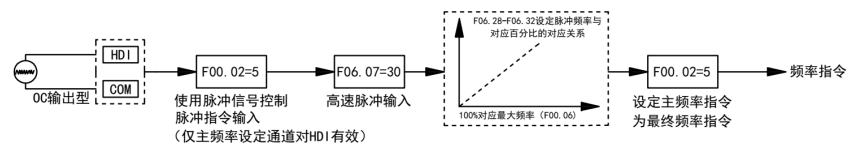
图 5-9 脉冲给定输入主频率参数设置
