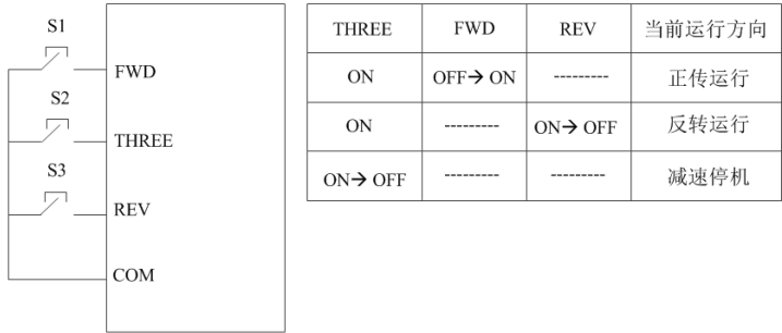
图 5-4 三线式控制 2
