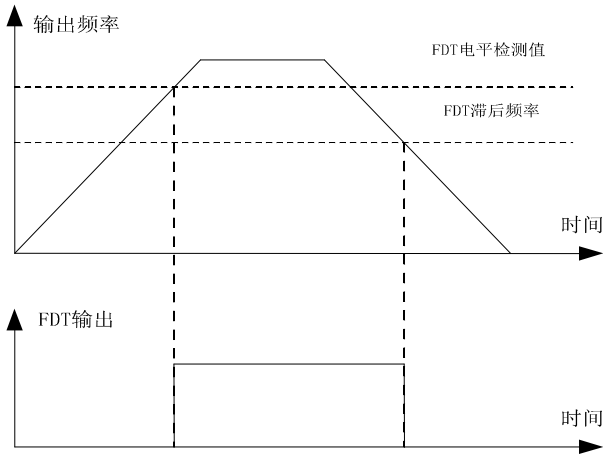
图 5-17 输出频率与 FDT 输出关系图
