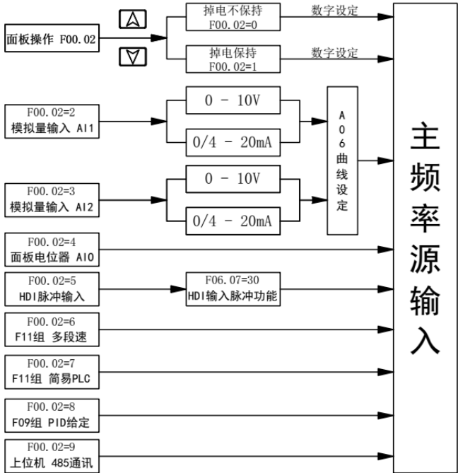
图 5-5 频率指令输入
