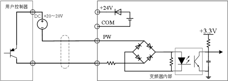
图 2-10 PNP 型拉电流接线方式
