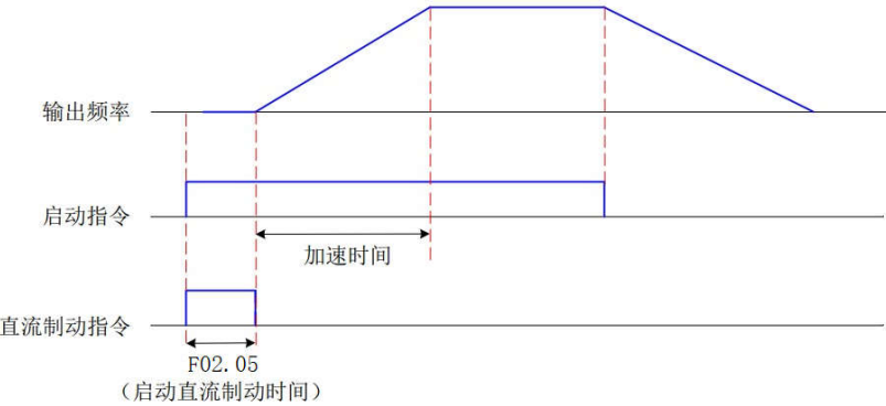
图 5-15 带直流制动的启动时序图
