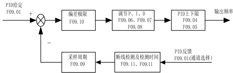
图 5-11 PID 控制原理
