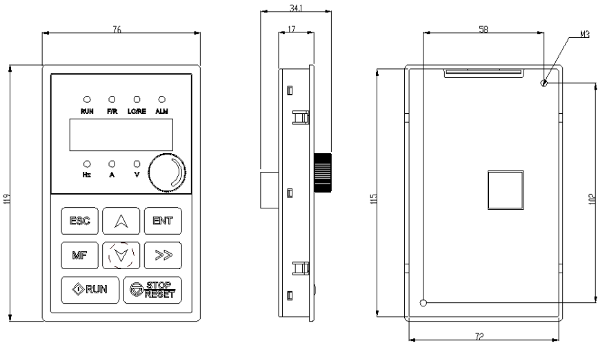
图 1-3 面板外形及尺寸图(单位 mm)
