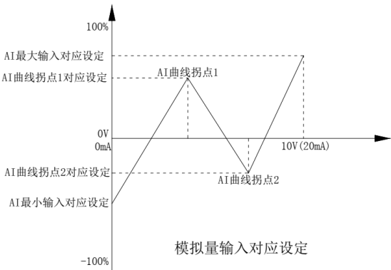
图 5-8 曲线 4 和曲线 5 设定示意图
