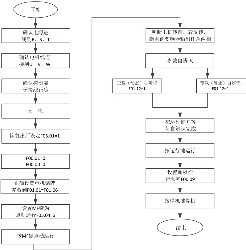
图 3-3 首次上电流程图
