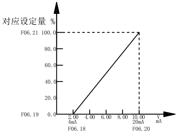
图 5-7 AI2 曲线设定示意图
