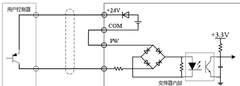
图 2-8 PNP 型拉电流接线方式
