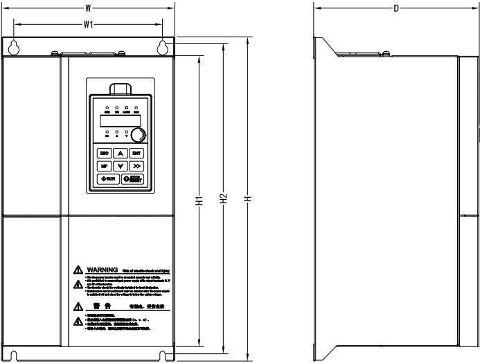
c) 适用于 C3~C6 机箱
