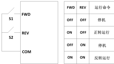
图 5-2 两线式控制 2
