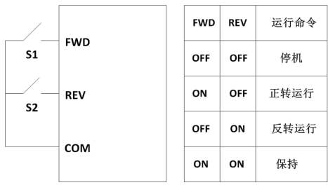
图 5-1 两线式控制 1
