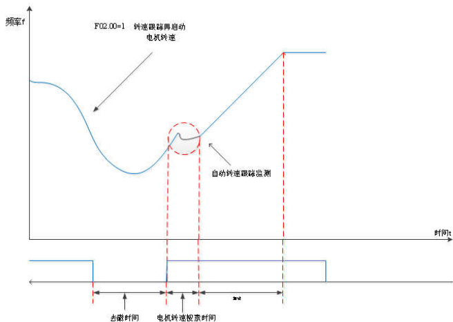
图 5-16 转速跟踪再启动方式
