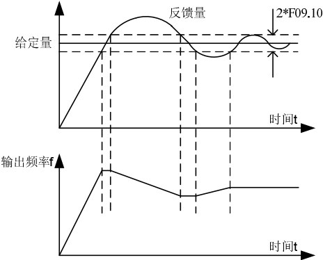
图 5-12 过程 PID 控制示例
