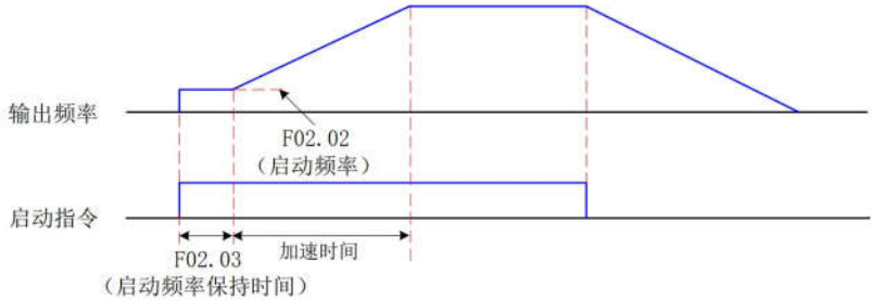
图 5-14 带启动频率的启动时序图
