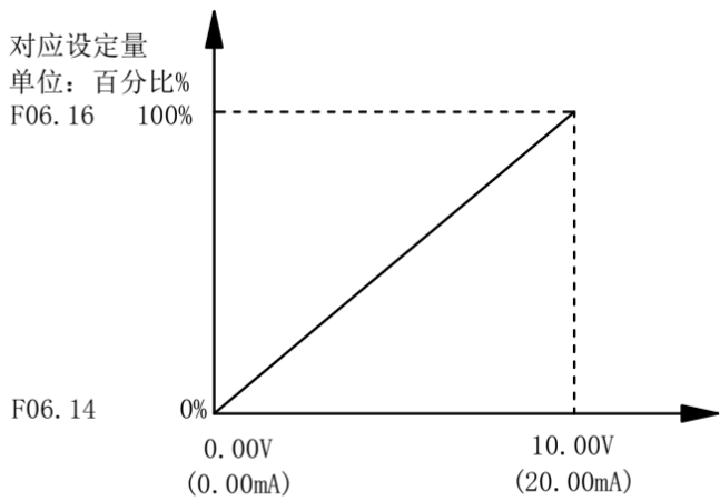
图 5-6 AI1 曲线设定示意图
