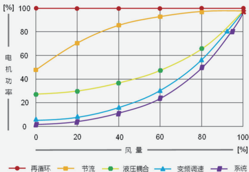
风机负载控制方式耗能对比
