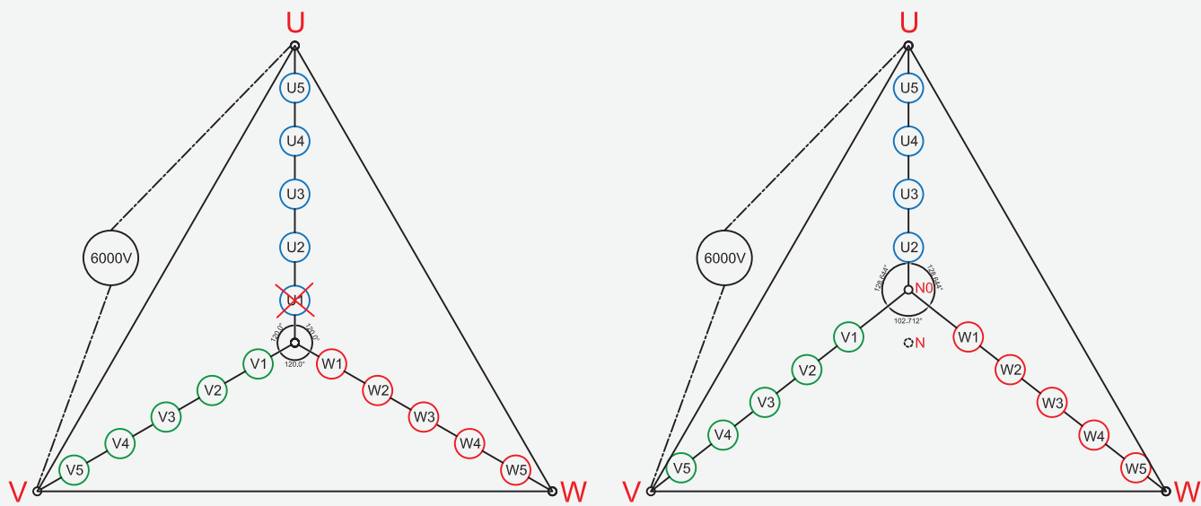
单元旁路电压向量图
