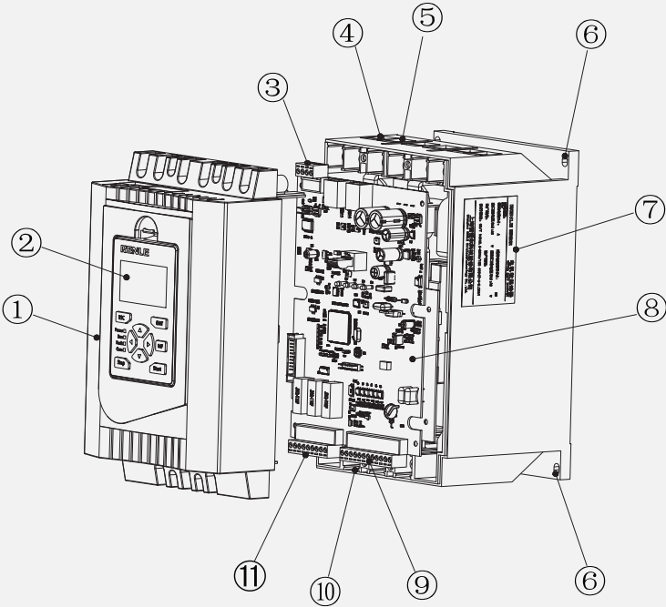
01 M0 产品结构布局
