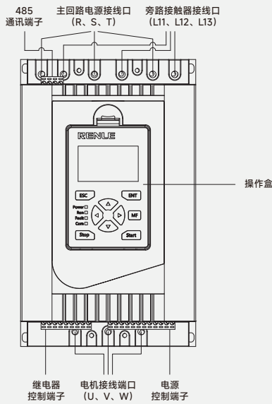
① 结构类型 M0 外形接线说明：
