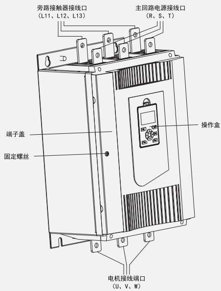
② 结构类型 M1-M3 外形接线说明：
