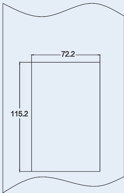
b) 面板本体开孔尺寸图
