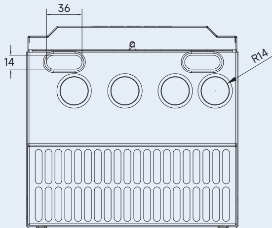
a) 适用于 RNB1015G/018P (含) ~ RNB1022G/030P(含)
