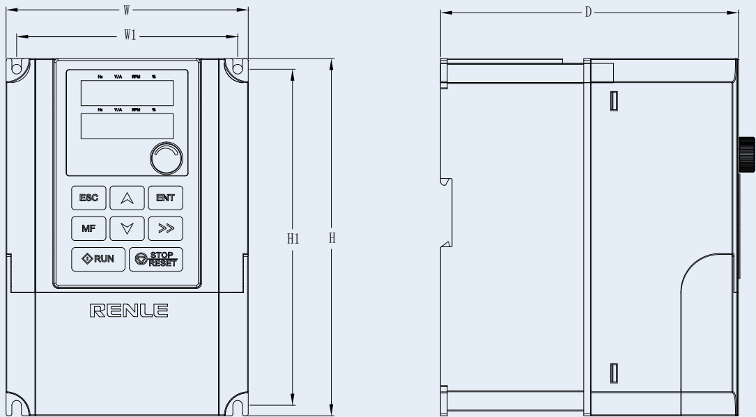
a) 适用于 RNB1000G (含) ~ RNB1004G/005P (含)
