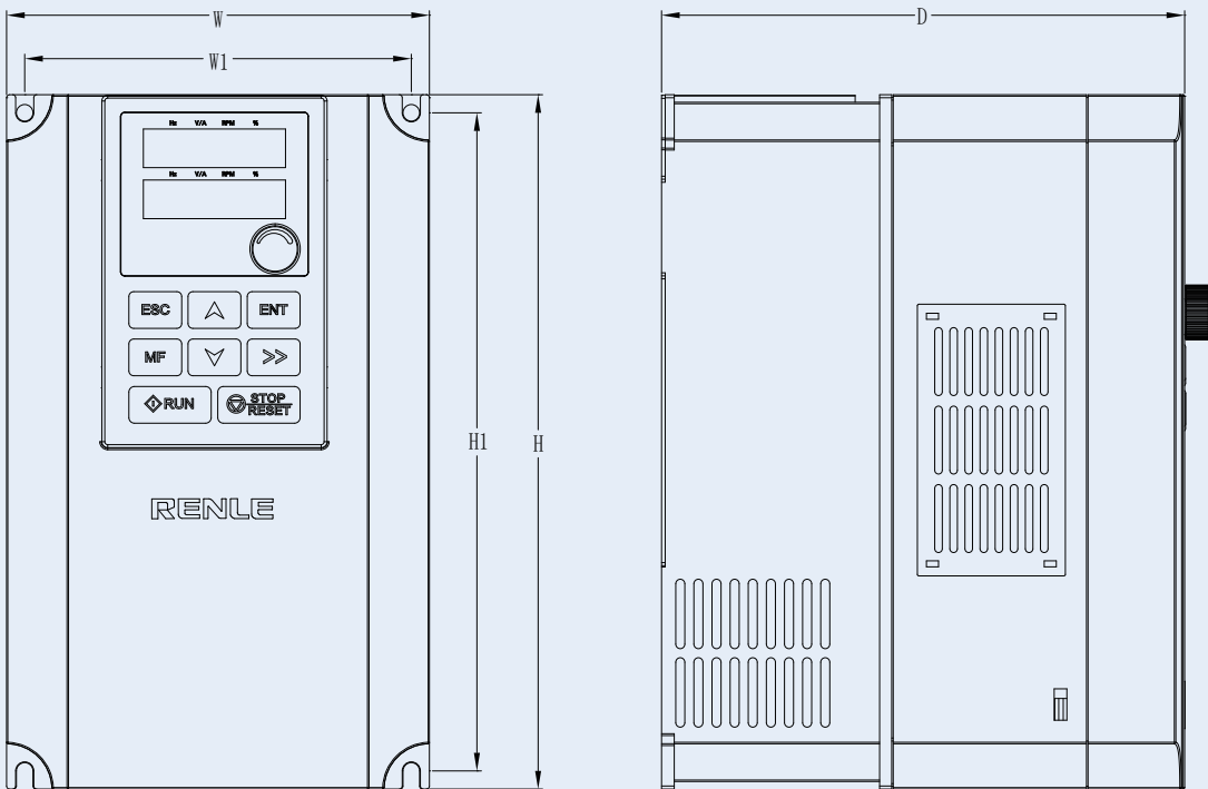
b) 适用于 RNB1005G/007P (含) ~ RNB1011G/015P (含)
