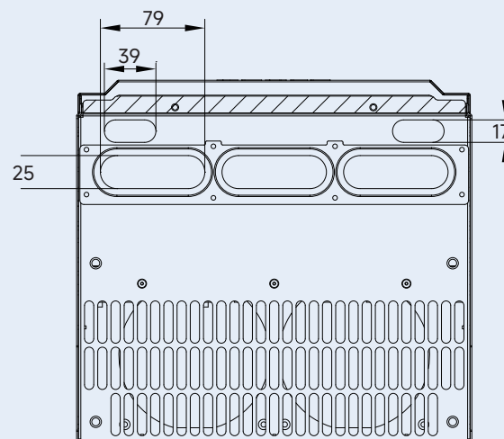
c) 适用于 RNB1045G/055P(含) ~ RNB1090G/110P(含)
