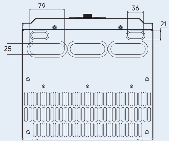
b) 适用于 RNB1030G/037P (含) ~ RNB1037G/045P(含)
