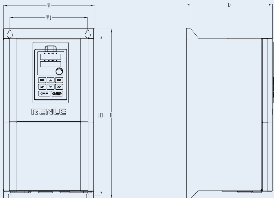
c) 适用于 RNB1015G/018P(含) ~ RNB1132G/160P(含)
