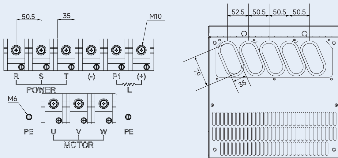
d) 适用于 RNB1110G/132P( 含 ) ~ RNB1132G/160P( 含 )
