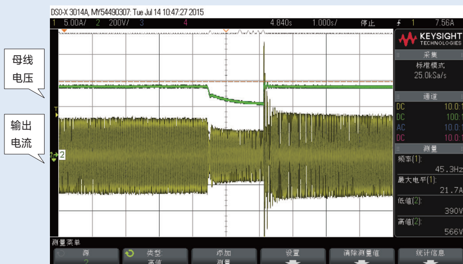
欠电压调节
