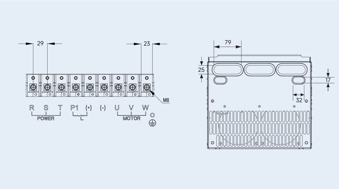
c) 适用于 RNB6045A ~ RNB6090A
