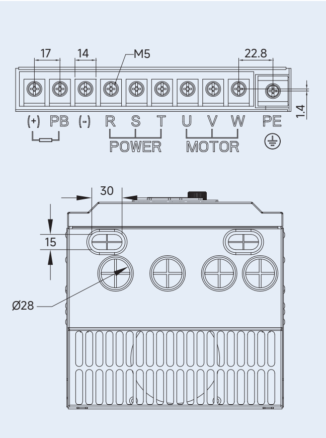
a) 适用于 RNB6015A ~ RNB6022A
