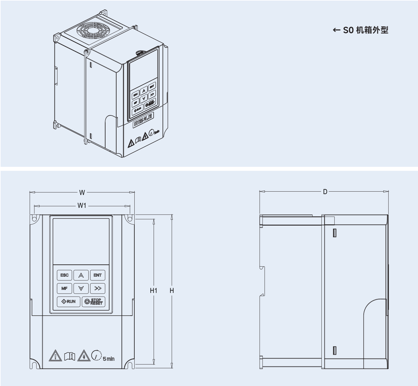
a) 适用于 RNB6001A ~ RNB6004A
