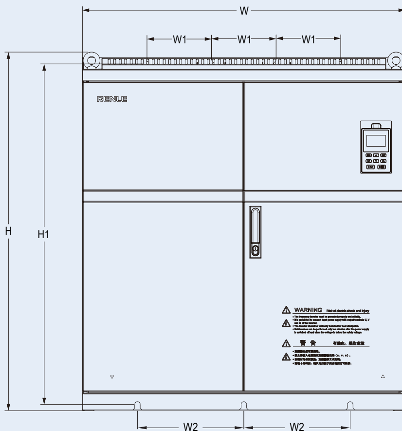
e) 适用于 RNB6450A ~ RNB6500A
