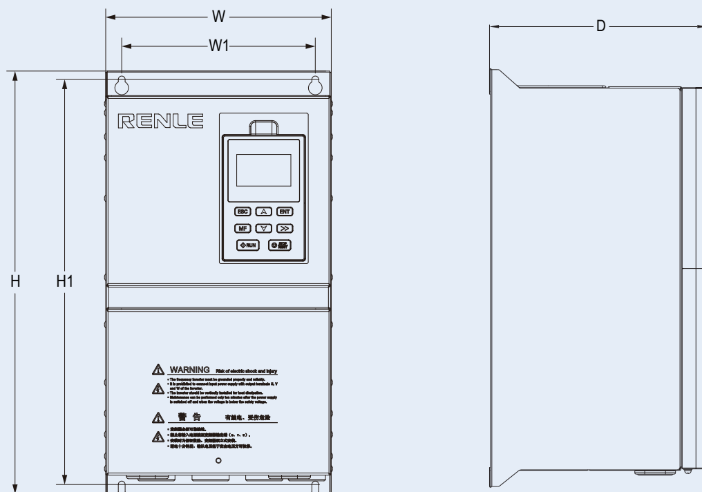
c) 适用于 RNB6015A ~ RNB6132A
