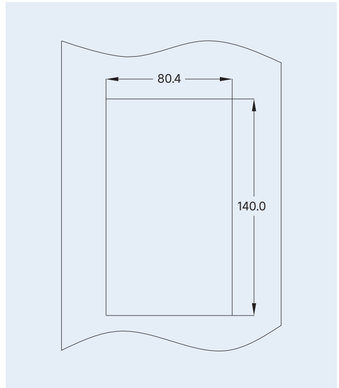
d) 面板支架开孔尺寸图
