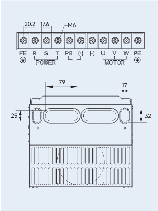
b) 适用于 RNB6030A ~ RNB6037A
